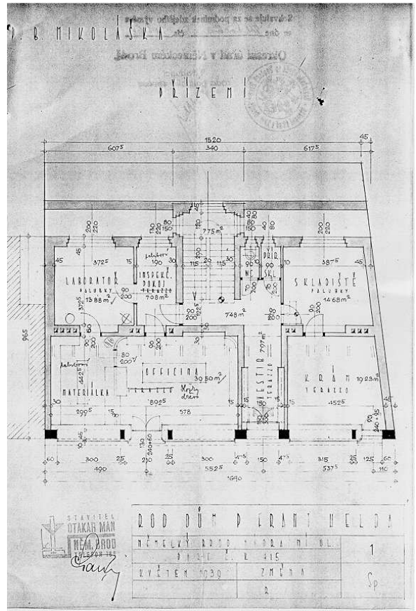
Příloha H2: Plán lékárny v domě čp.606, přízemí.
