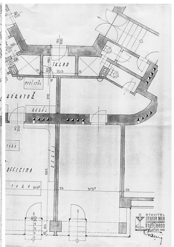
Příloha H2: Plán lékárny v domě čp.606, přízemí.
