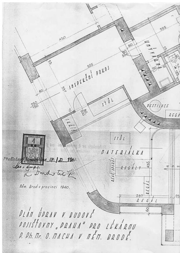
Příloha H3: Plán lékárny v domě čp.582
