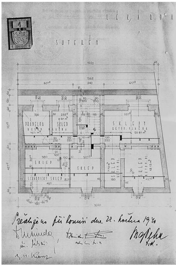
Příloha H2: Plán lékárny v domě čp.606, suterén.
